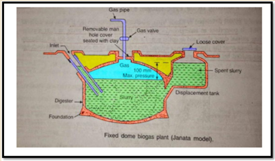
الشكل ذو العدد (٤): مخمر جانتا
