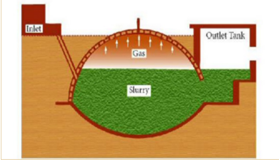
الشكل ذو العدد (٧): مخمر دينباندھو
