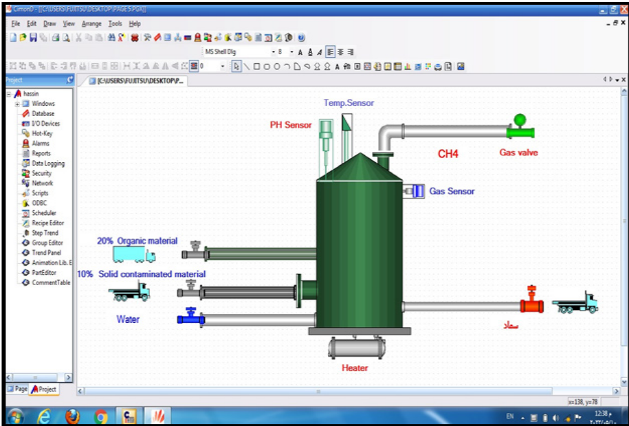
الشكل ذو العدد (١٦) منظومة الهاضم الحيوي مع عملية السيطرة
